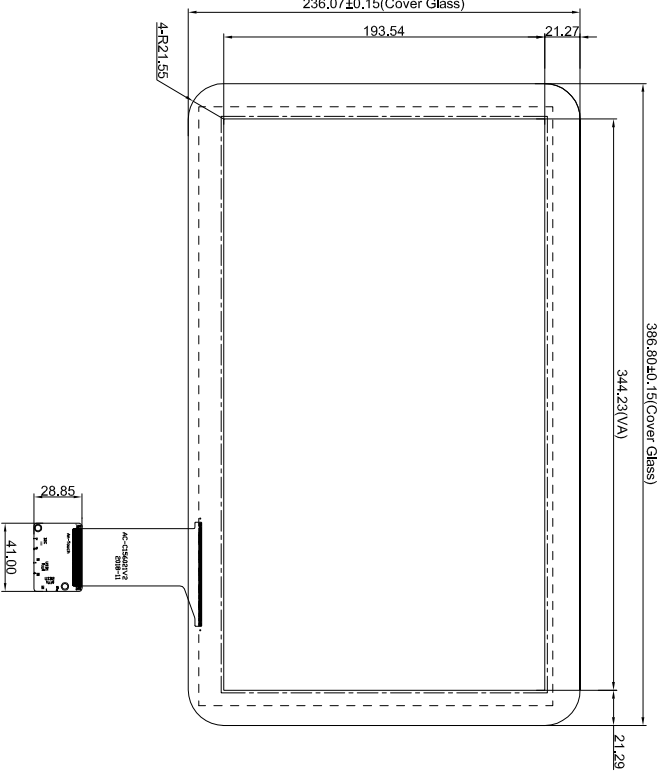
正视图
