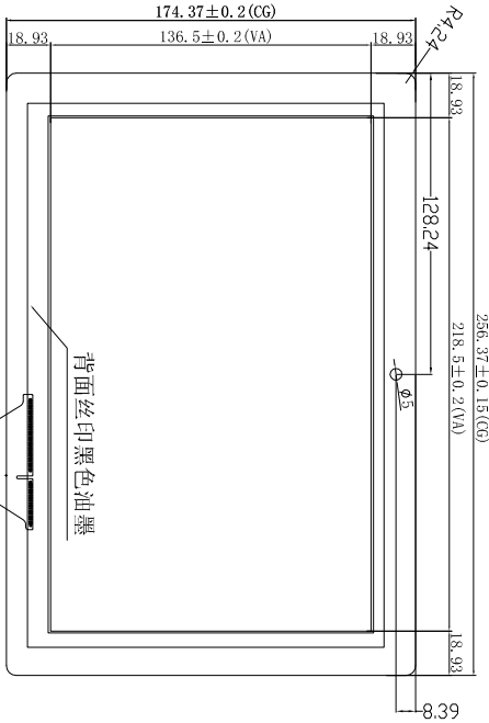
正视图
