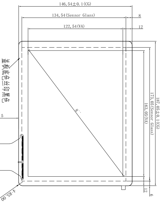
正视图
